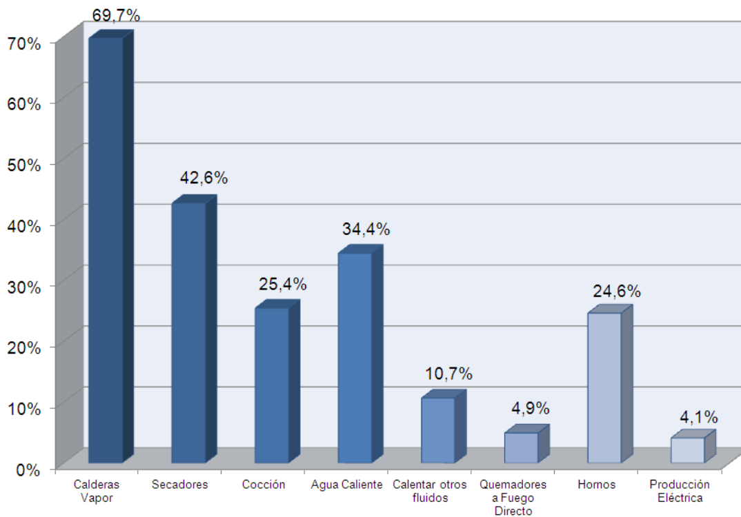
Figura 9. Frecuencia de aplicaciones relacionadas de energía térmica en PyME
